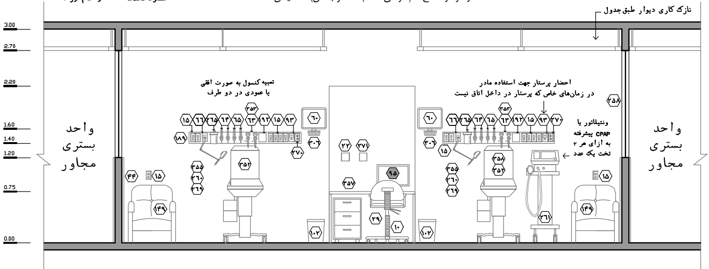
نقشه ۲-۴۳- نمای ۱- مقیاس ۱:۵۰
