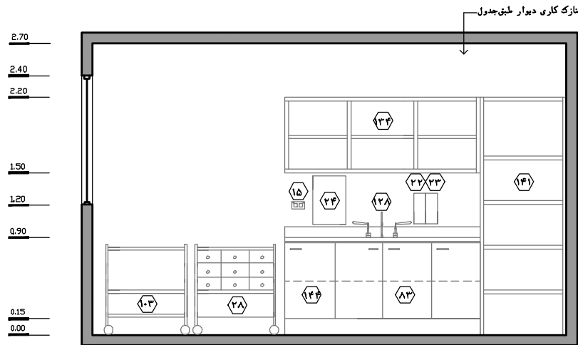
نقشه‌ی ۸۲-۲-۲- نمای ۲- مقیاس ۱:۵۰
