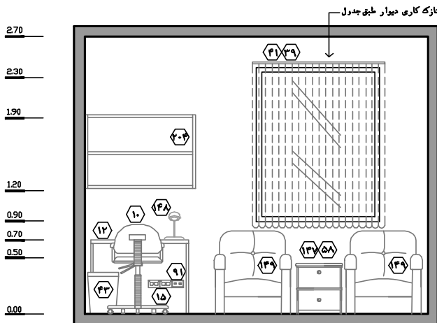
نقشه‌ی ۲-۱۰۸-۱- نمای ۲ - مقیاس ۱:۵۰
