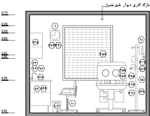
نقشه‌ی ۲-۵۷ - نمای ۳ - مقیاس ۱:۵۰
