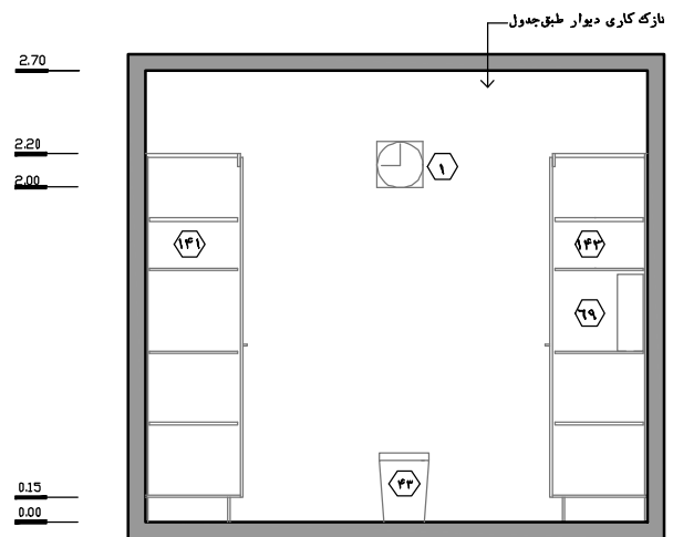
نقشه‌ی ۸۴-۲-۴- نمای ۴- مقیاس ۱:۵۰
