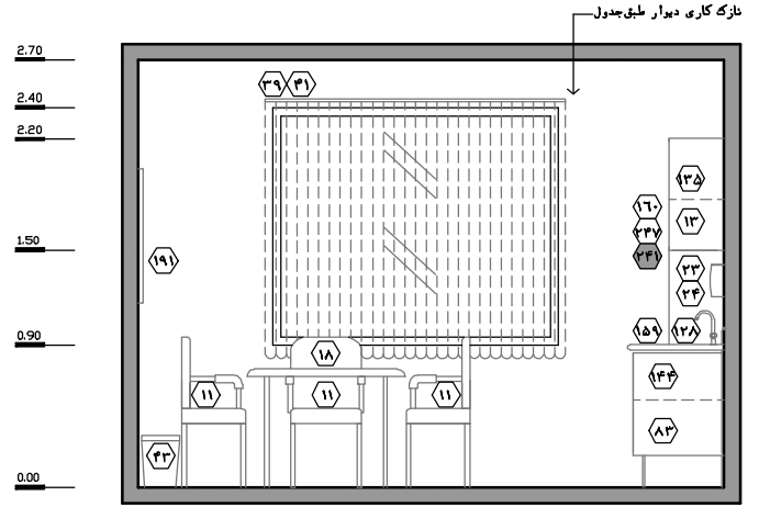
نقشه‌ی ۲-۱۱۳- نمای ۳- مقیاس ۱:۵۰
