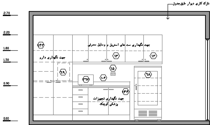
نقشه‌ی ۸۱-۲-۱- نمای ۱- مقیاس ۱:۵۰
