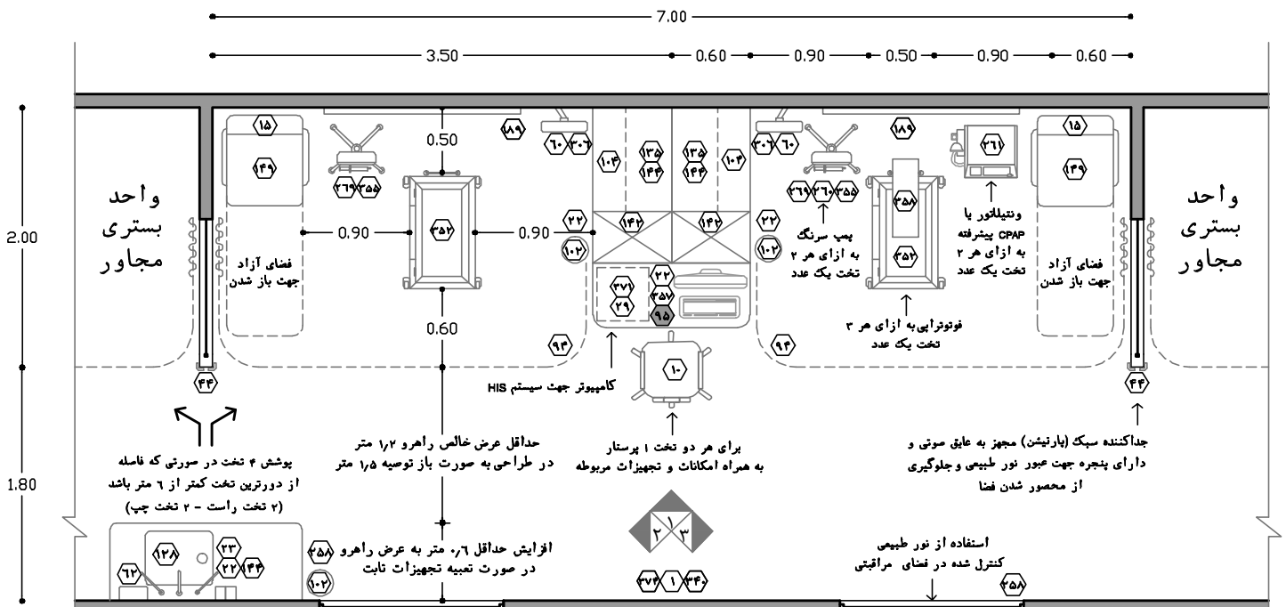
نقشه ۲-۴۳- پلان نمونه‌ی فضای باز بستری در بخش مراقبت‌های ویژه نوزادان در مراکز سطح ۳ (طراحی ادغام‌شده دو بخش) - مقیاس ۱:۵۰
