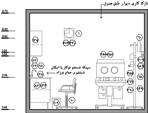
نقشه‌ی ۲-۶۰-۲- نمای ۲- مقیاس ۱:۵۰
