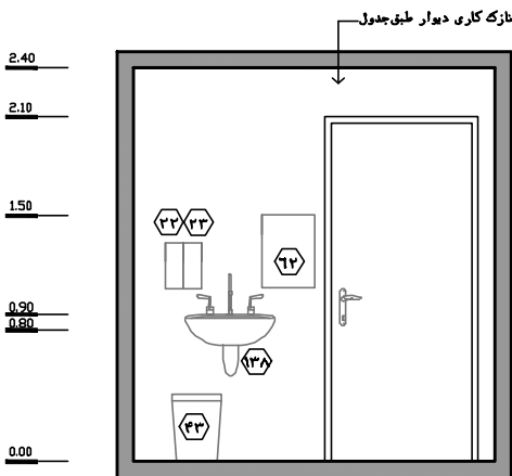
نقشه ۲-۱۱۸- نمای ۱- مقیاس ۱:۵۰
