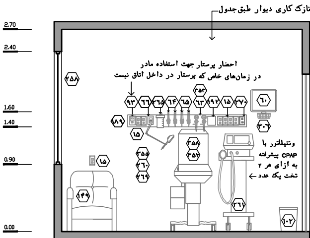
نقشه‌ی ۲-۵۵ - نمای ۱ - مقیاس ۱:۵۰
