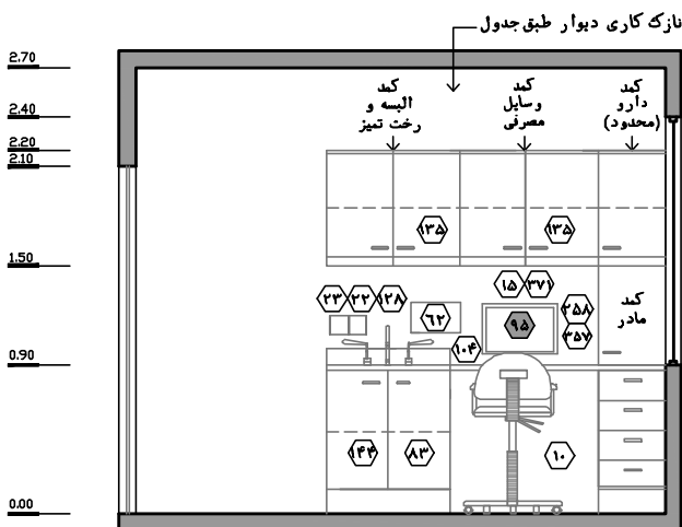
نقشه‌ی ۲-۵۶ - نمای ۲ - مقیاس ۱:۵۰
