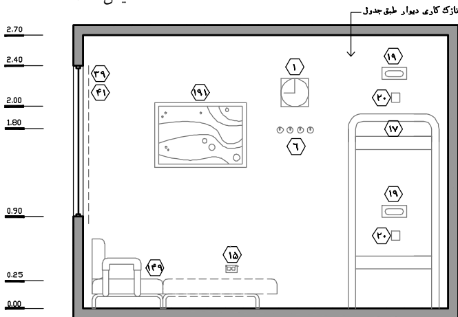
نقشه‌ی ۲-۱۰۷-۱- نمای ۱ - مقیاس
