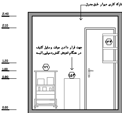
نقشه ۲-۱۲۰- نمای ۳- مقیاس ۱:۵۰
