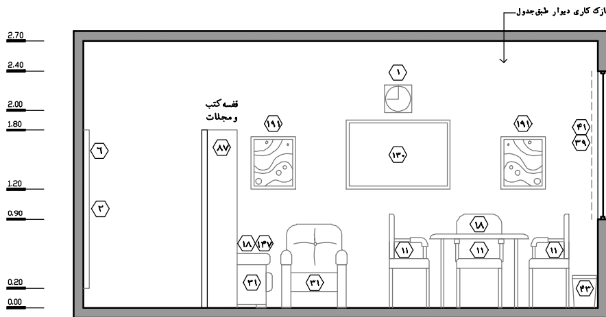
نقشه‌ی ۲-۱۱۴- نمای ۴- مقیاس ۱:۵۰
