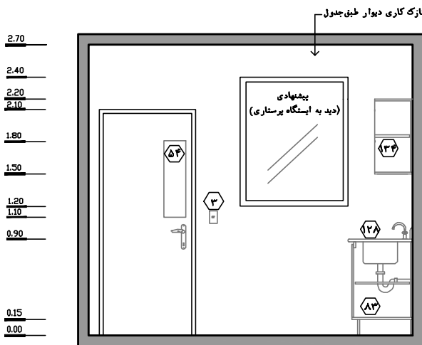
نقشه‌ی ۸۳-۲-۳- نمای ۳- مقیاس ۱:۵۰
