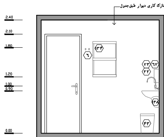
نقشه ۲-۱۱۹- نمای ۲- مقیاس ۱:۵۰
